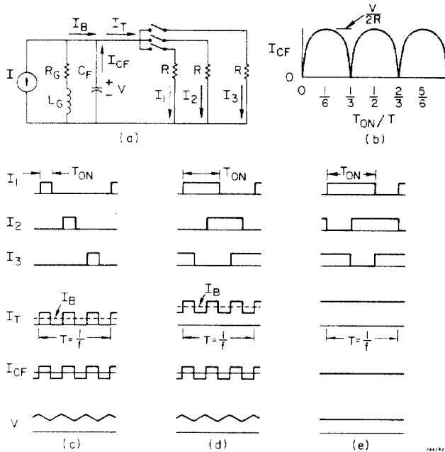
FIG. 3--(a) Idealized 3-phase chopper; (b) filter capacitor current; (c) T_{ON}/T=1/6 ; (d) T_{ON}/T=1/2 ; (e) T_{ON}/T=2/3 .
