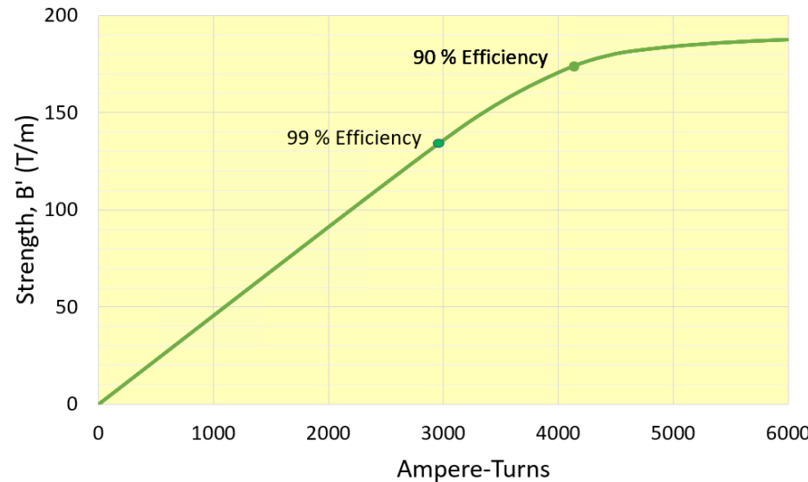
NSLS-IIU Quadrupole
