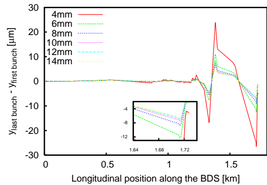
(b) 500 TeV
